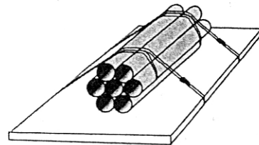
Xếp, cố định ống trụ nặng ngang thùng xe
