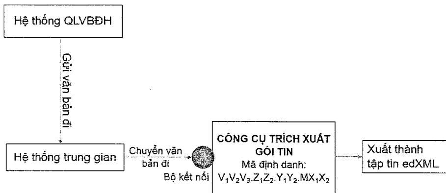
Hình B.2 - Sơ đồ ghép nối để trích xuất gói tin đi ra từ hệ thống trung gian
