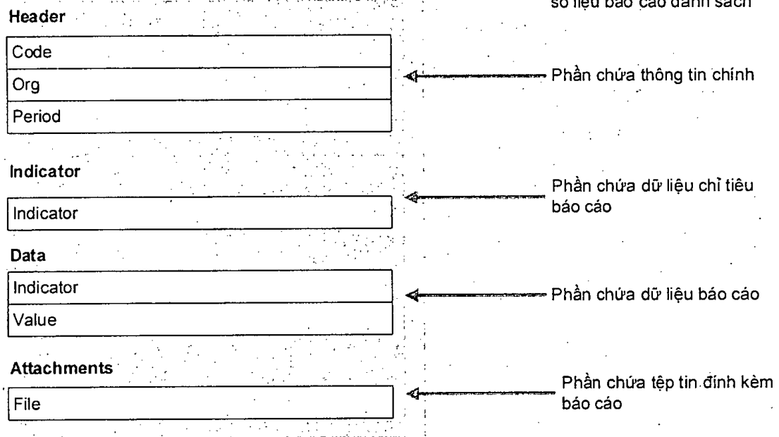
Hình 5 - Cấu trúc gói tin số liệu báo cáo danh sách
